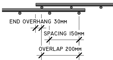
A Section A 1 : 10
